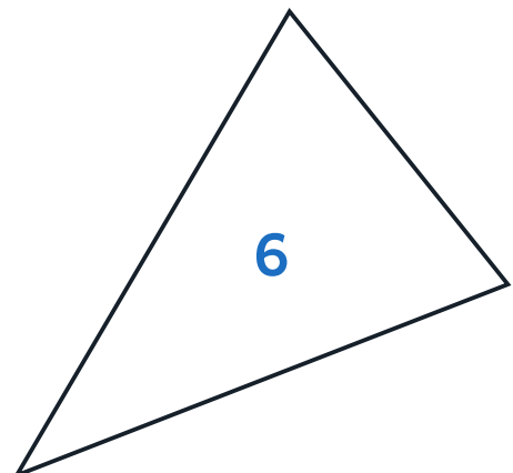
6. obtuse scalene
