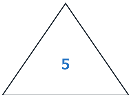
5. obtuse
